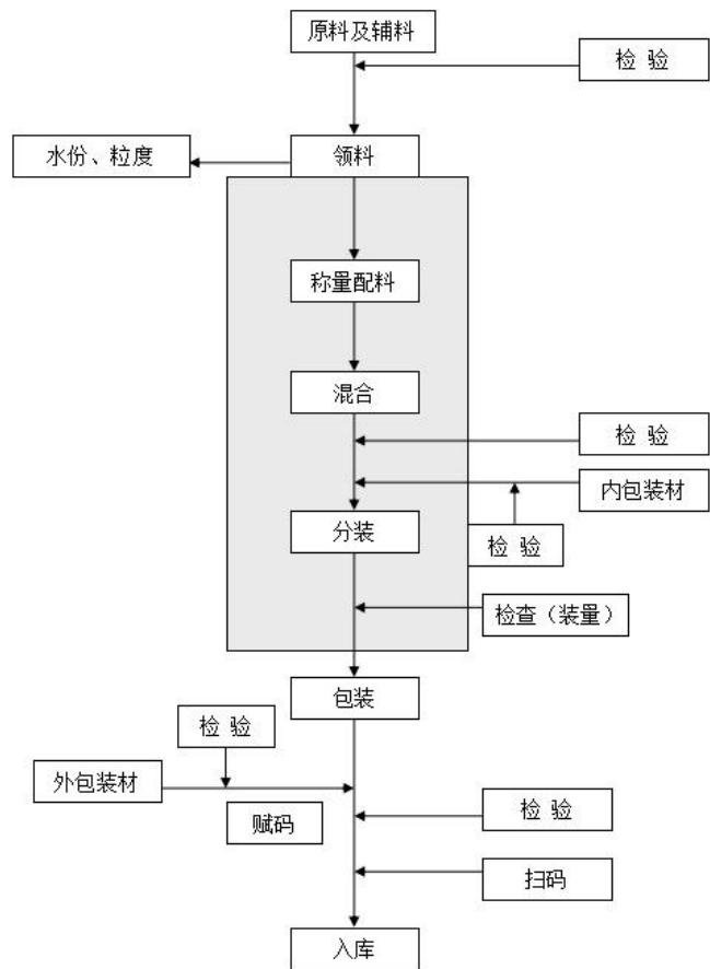
13-2 粉剂/预混剂工艺流程图
